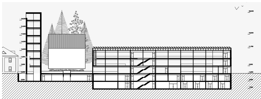
POZDĽŽNY REZ
