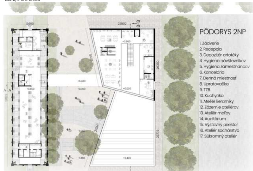
PÔDORYS 1. NADZEMNÉHO PODLAŽIA
