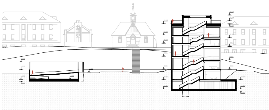
POZDĽŽNY REZ
