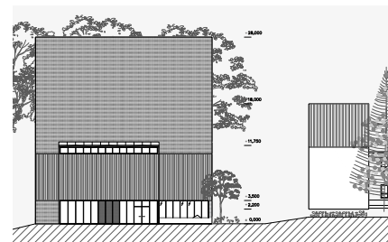
POHĽAD ZÁPADNÝ, VÝCHODNÝ
