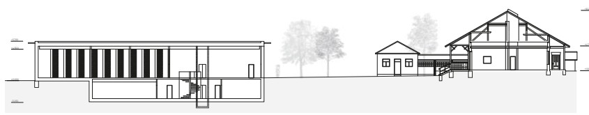
POZDĽŽNY REZ
