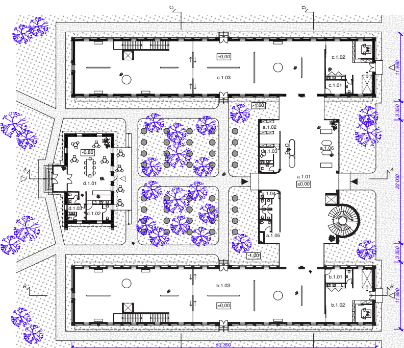
PÔDORYS 1. NADZEMNÉHO PODLAŽIA
