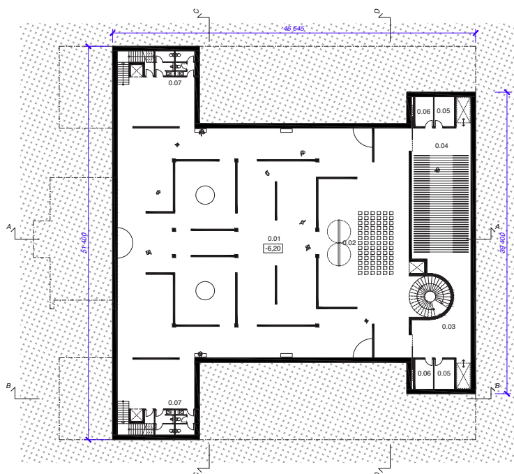
PÔDORYS 1. PODZEMNÉHO PODLAŽIA
