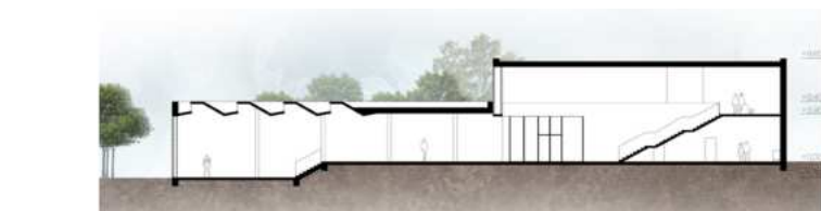
POZDĽŽNY REZ
